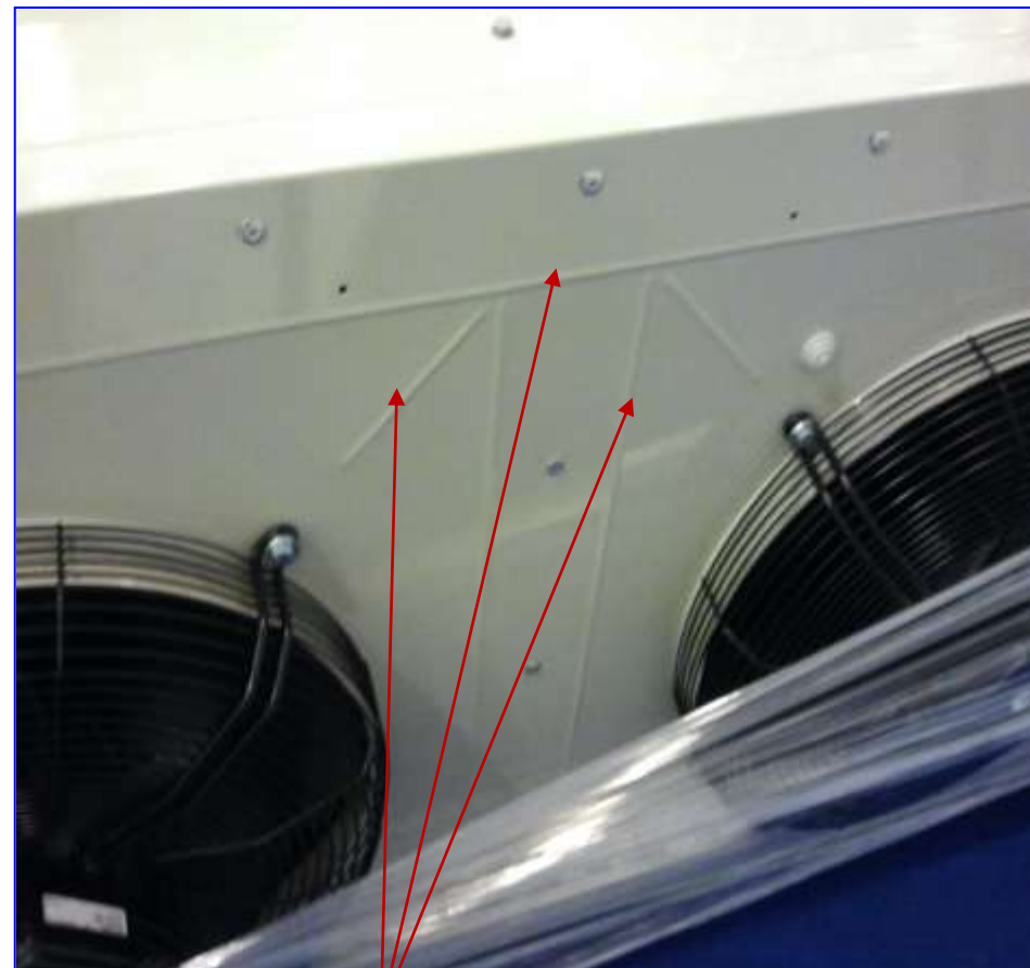
Наличие ребер жесткости при большей или равной толщине корпусного металла (FRITERM)
