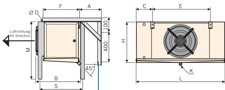
Wandkonsolen für Typen 045.2, 050.2 Стенная консоль для типов 045.2, 050.2
