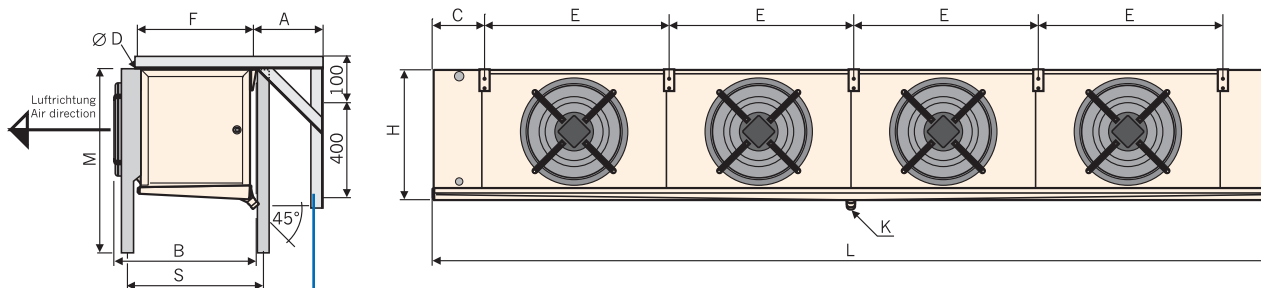
Wandkonsolen für Typen 045.2, 050.2 Стенная консоль для типов 045.2, 050.2
