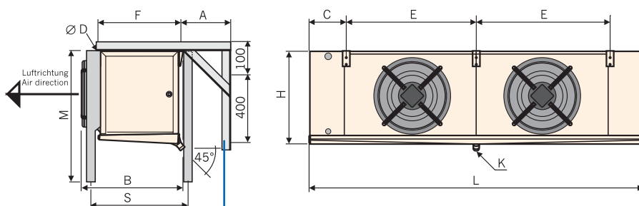
Wandkonsolen für Typen 045.2, 050.2 Стенная консоль для типов 045.2, 050.2
