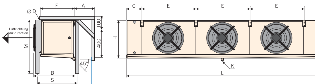
Wandkonsolen für Typen 045.2, 050.2 Стенная консоль для типов 045.2, 050.2
